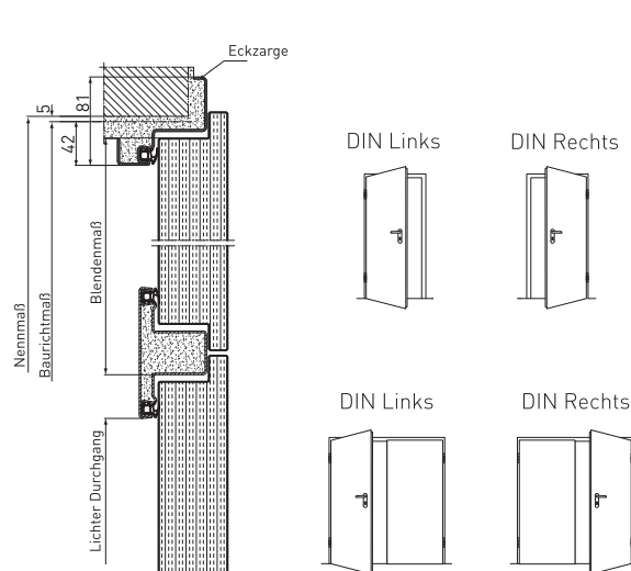
Vertikalschnitt mit Oberblende
