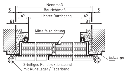
Horizontalschnitt 2-flgl.
