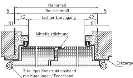
Horizontalschnitt 2-flg.
