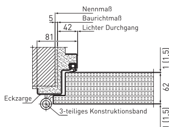
Horizontalschnitt 2-flgl.
