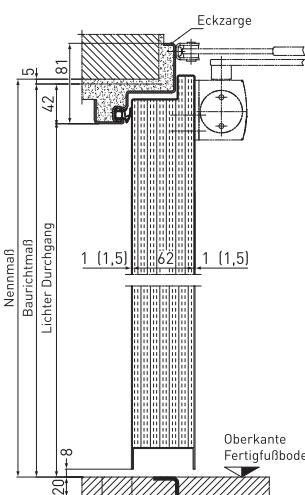
Vertikalschnitt
