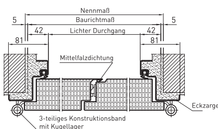
Horizontalschnitt 2-flgl.
