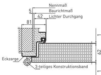
Horizontalschnitt 2-flgl.
