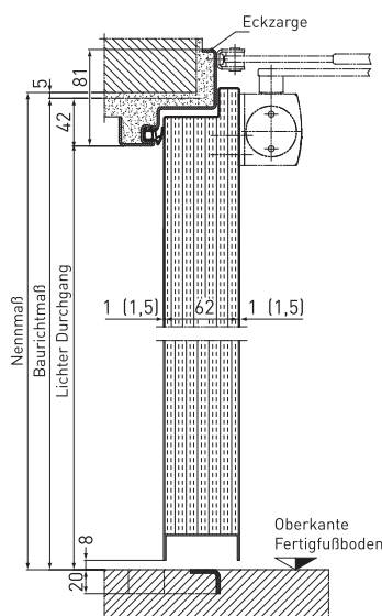
Vertikalschnitt
