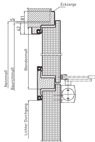
Vertikalschnitt mit Oberblende
