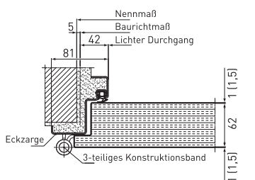
Horizontalschnitt 2-flg.
