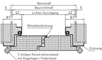
Horizontalschnitt 2-flgl.
