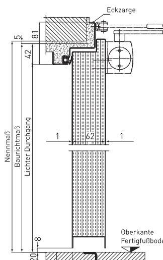
Vertikalschnitt
